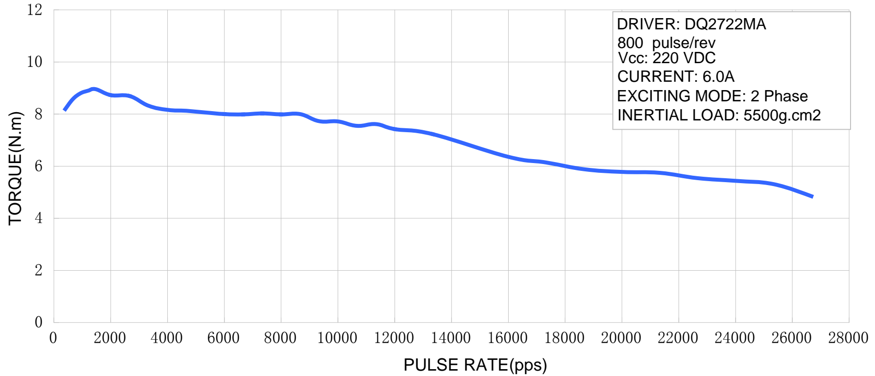
110BYGH99-001 Torque Curve
